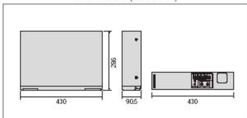
Dimensions (unit : mm)
